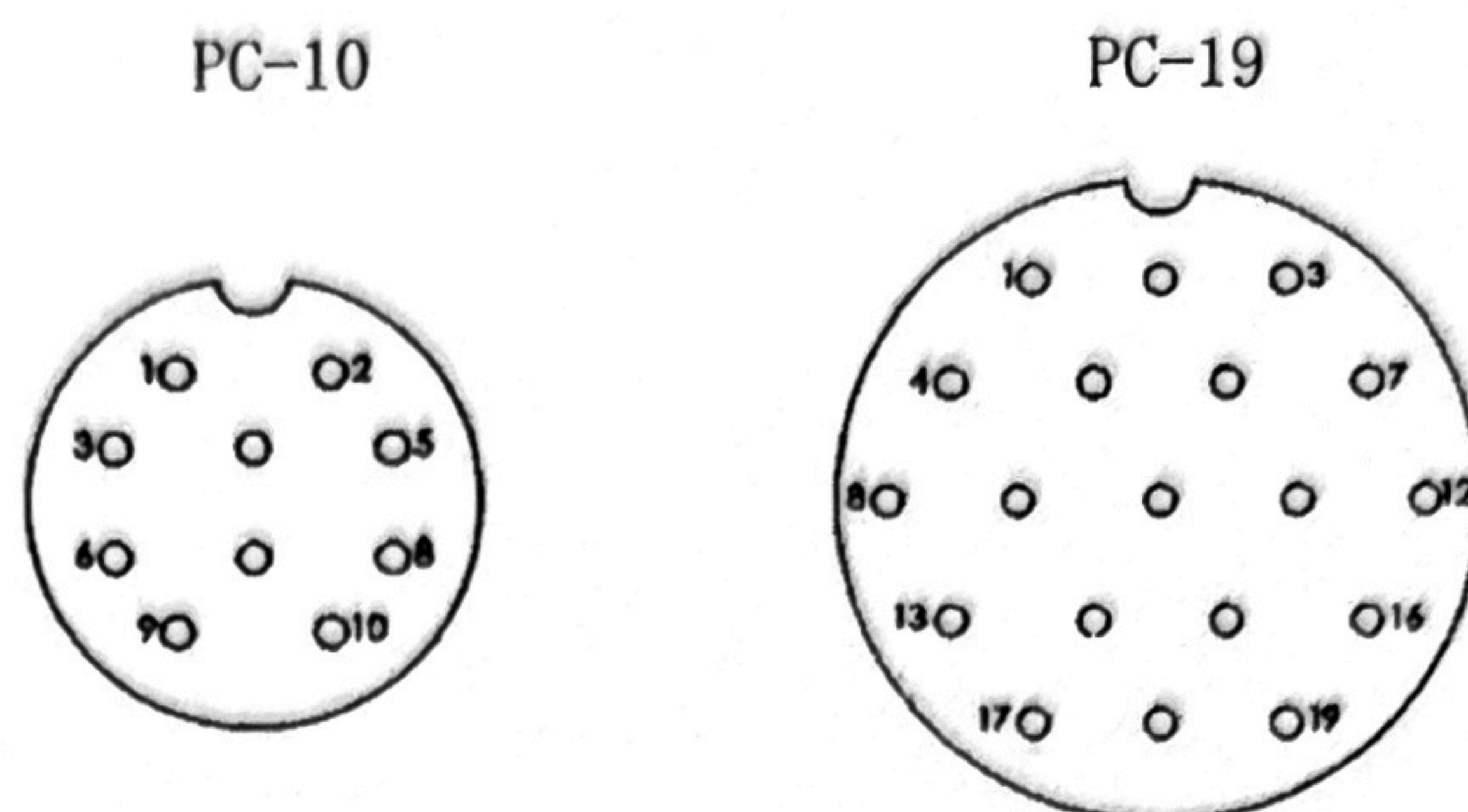
图 1 绝缘体孔组排列
